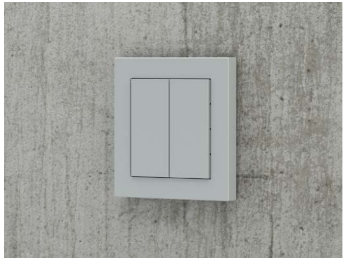
E12 – vypínač s měřením teploty Provedení Fenix NTM, efeso šedá, červená/bílá LED Rozměry: 87 × 87 × 9 mm Vnitřní hmatníky 60 × 60 mm
